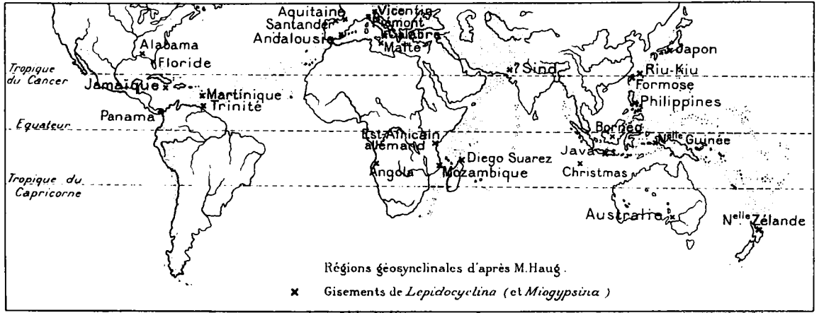
Fig. 4. — Carte de la répartition géographique des Lepidocyclines .
