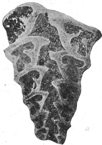
Fig. 4. — Nerinea Renauxiana D'ORB. — Section grand. naturelle.
