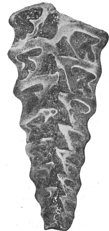
Fig. 3. — Nerinea Coquandiana D'ORB. — Section grand. nat.
